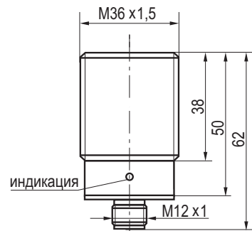
Габаритный чертеж
